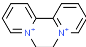
Diquat
